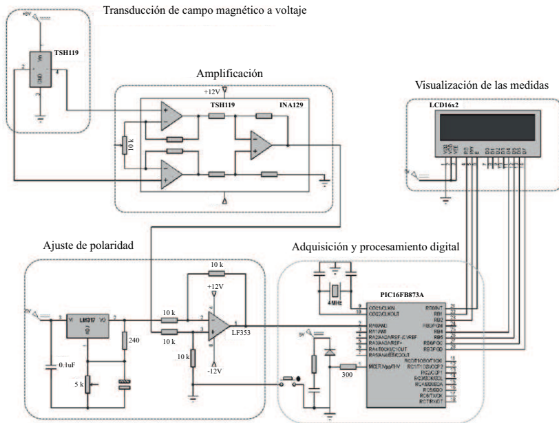
Figura 6: Esquema del circuito electrónico del teslámetro, diferenciando los diferentes módulos.
