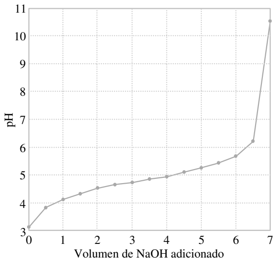
Titulación ácido débil base fuerte Volumen adicionado vs pH
