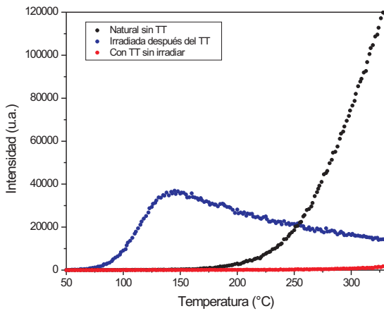
Figura 2: espectros TL de arena natural sin tratamiento térmico (TT), con un TT de 400°C por una hora y después de recibir una irradiación de 50 cGy
