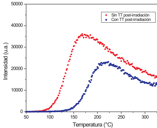
Figura 4: espectro TL para una muestra de la playa de Coveñas irradiada a una dosis de 50 cGy y sometida a un tratamiento térmico post-irradiación de 100°C por diez minutos
