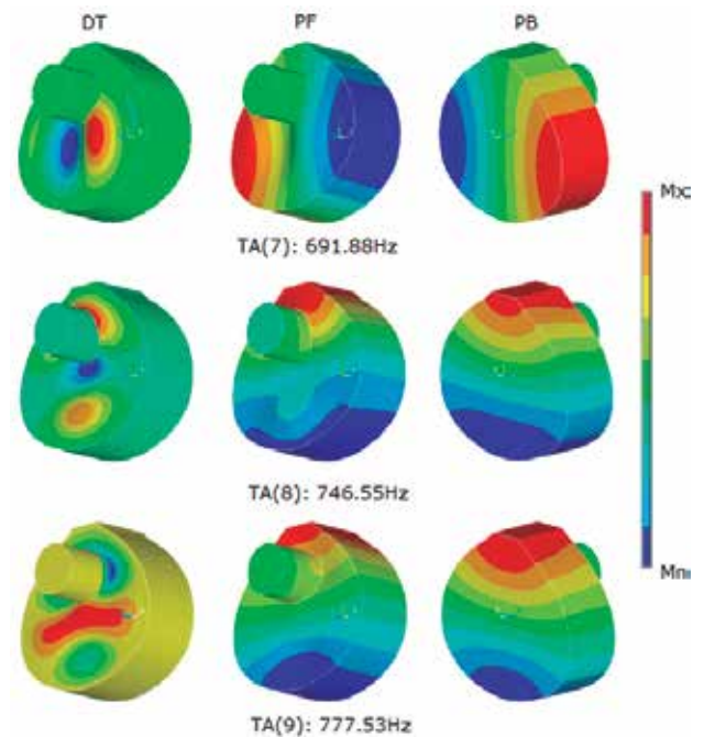
Figura 13. Modos normales de vibración acoplados, del sistema placa frontal-aire encerrado. Modos 7-9.
