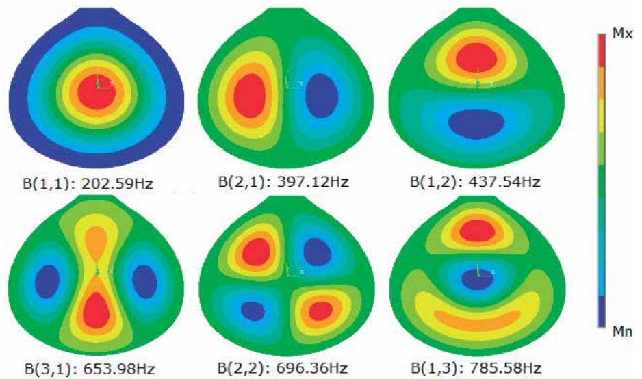
Figura 9. Modos normales de vibración de la placa posterior de la bandola en un rango de 0-800 Hz.
