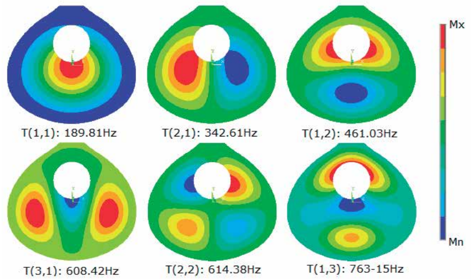
Figura 8. Modos normales de vibración de la placa frontal de la bandola en un rango de 0-800 Hz.
