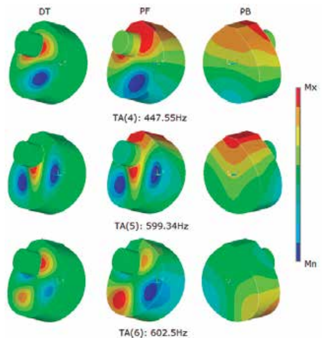
Figura 12. Modos normales de vibración acoplados, del sistema placa frontal-aire encerrado. Modos 4-6.
